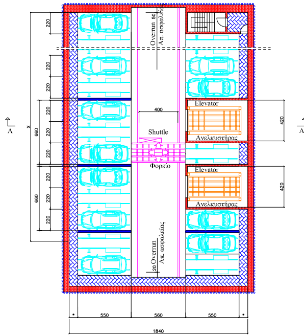
Typical floor plan Τυπικός όροφος
