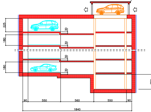
Cross section A-A Τομή A-A
